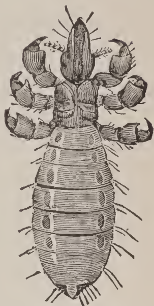
FIG. 550. — Hog-louse.
