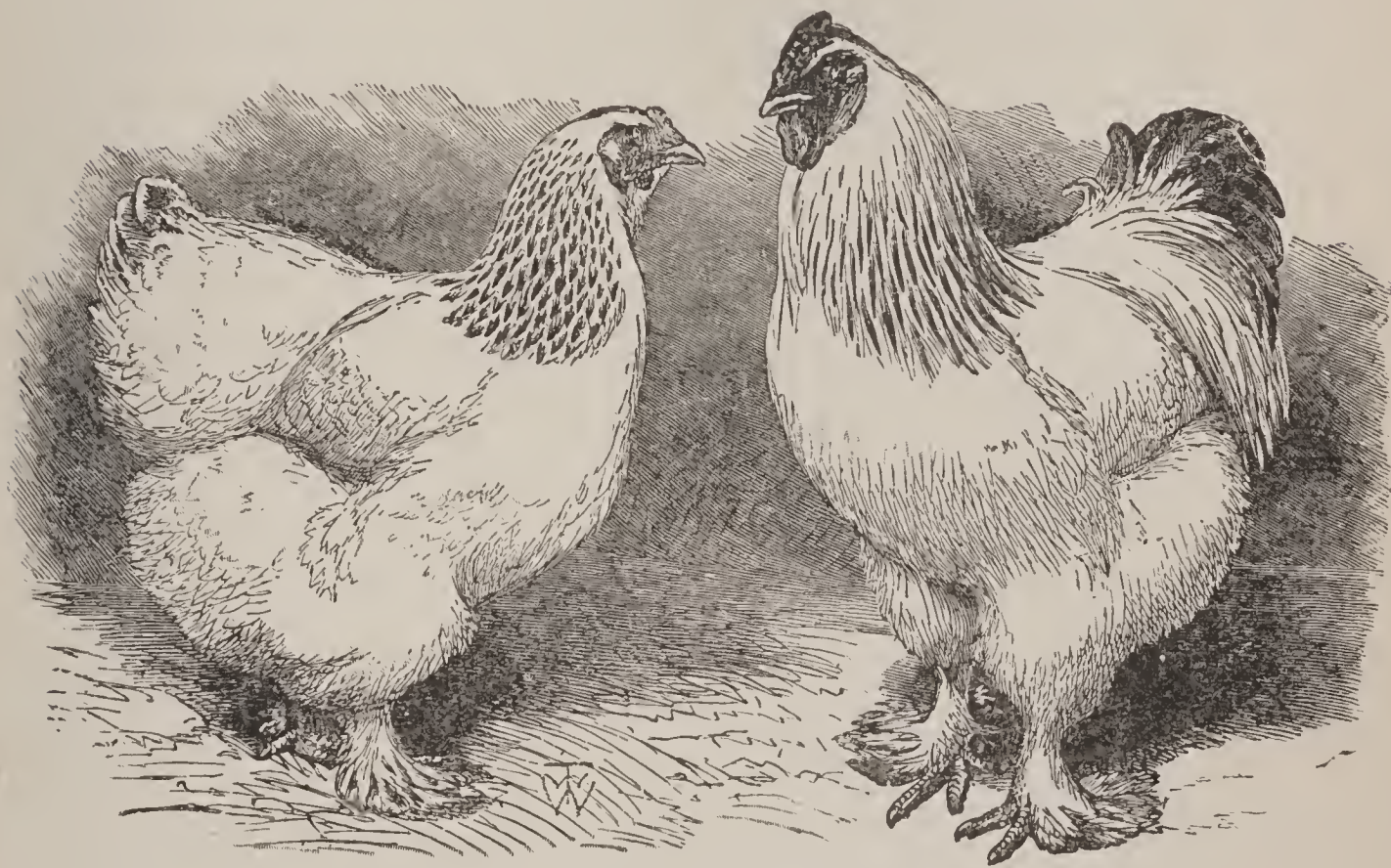
FIG. 555. — Light brahmas.
