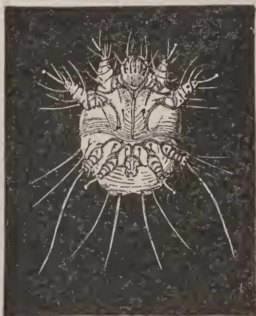
FIG. 282. — Mange parasite.
