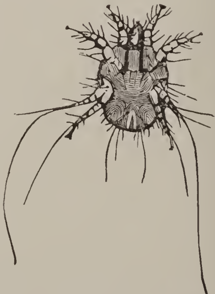
FIG. 280. — Mange parasites.
